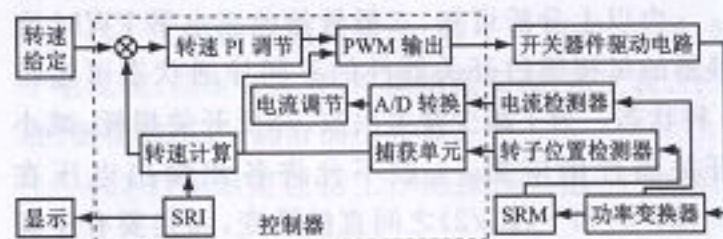
图1 开关磁阻电动机调速系统组成框图
